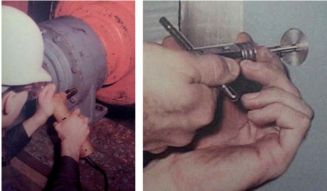
孔口平面，转孔后攻螺纹
