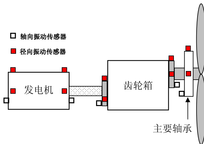
带有加速度振动传感器的水平布置的风力发电机组
